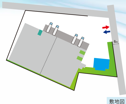
敷地図
